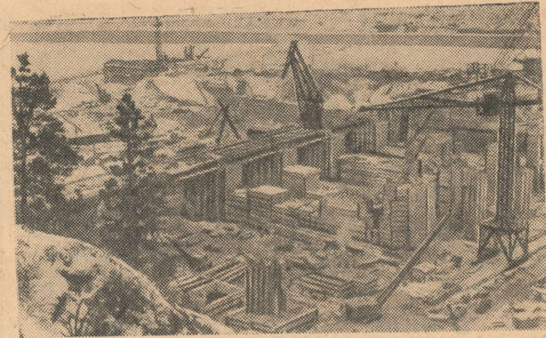
КРАСНОЯРСКИЙ КРАЙ. Строители будущего гиганта энергетики — Красноярской ГЭС готовятся к перекрытию Енисея. На плотине гидроэлектростанции круглые сутки ведутся бетонные работы.
