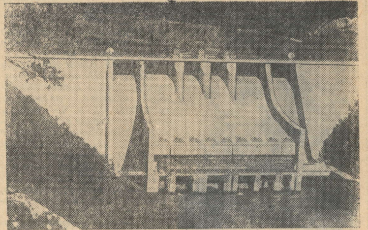
НАРОДНАЯ РЕСПУБЛИКА БОЛГАРИЯ. Плотина гидроэлектростанции Ивайловград, сооруженная в Родопских горах на реке Арда. Ее длина 250 метров, высота — 70 метров. Созданное здесь водохранилище объемом свыше 180 миллионов кубометров воды, позволяет орошать не только большие площади плодородных родопских полей, но и 30 тысяч гектаров земельных угодий в Греции.
