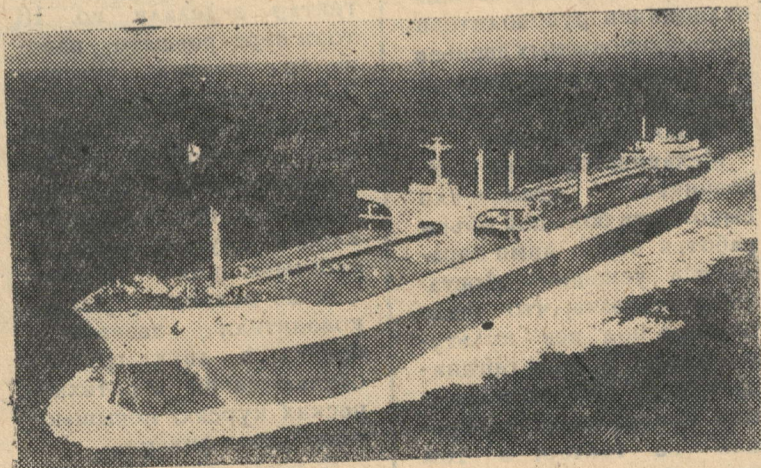
Крупнейший в мире танкер „Идэмицу-мару“ отправился в свой первый рейс в Кувейт. Уникальное судно водоизмещением 210 тысяч тонн, длиной 342 метра, шириной почти 50 метров построено в Японии. Управление гигантом полностью автоматизировано, команда состоит из 32 человек.
