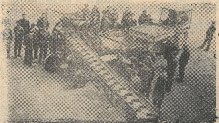
ЭСТОНСКАЯ ССР. Тартуский завод сельскохозяйственных машин «Выйг» приступил к изготовлению транспортеров-загрузчиков ТЗК-30, работающих при помощи электроэнергии. Машины предназначены для погрузки картофеля, их производительность 30 тонн в час. В этом году завод изготовит 250 таких транспортеров.
