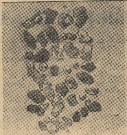
* Образец лунного грунта, доставленного автоматической станцией «Луна-16». На снимке слева — частицы разных горных пород в составе лунного реголита (раздробленной породы). Увеличено.
