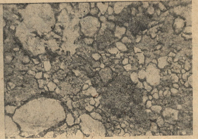
Справа — крупнозернистая часть нижней зоны колонки лунного грунта, доставленного автоматической станцией «Луна-16».
