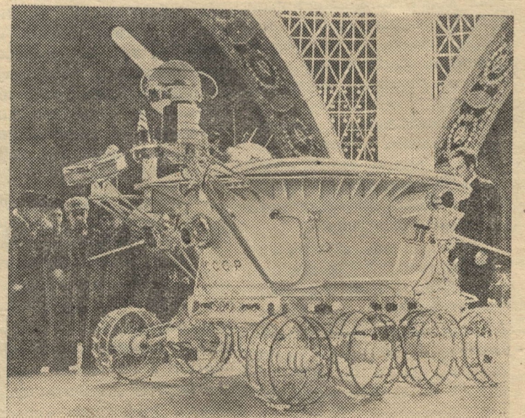
МОСКВА. Экспозиция павильона «Космос» Выставки Достижений Народного Хозяйства СССР пополнилась новым уникальным экспонатом. Здесь установлена точная копия первой передвижной автоматической лаборатории «Луноход-1» для комплексного изучения особенностей строения лунной поверхности, окололунной среды и дальних космических объектов. Фотохроника ТАСС.
