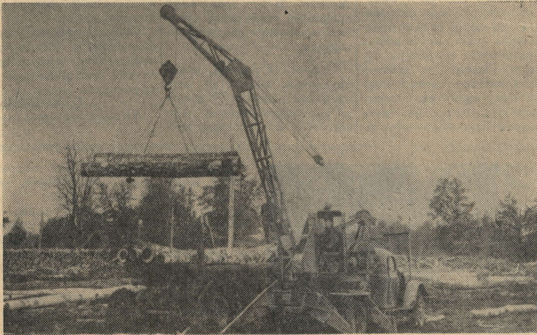
На этом снимке вы видите механизированную погрузку автокраном фанерного сырья на сортиментный лесовоз в пос. Бутаиха. Фото М. Каризина.
