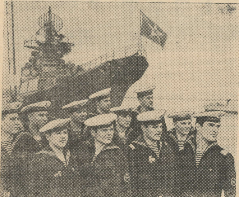
Фотохроника ТАСС.
